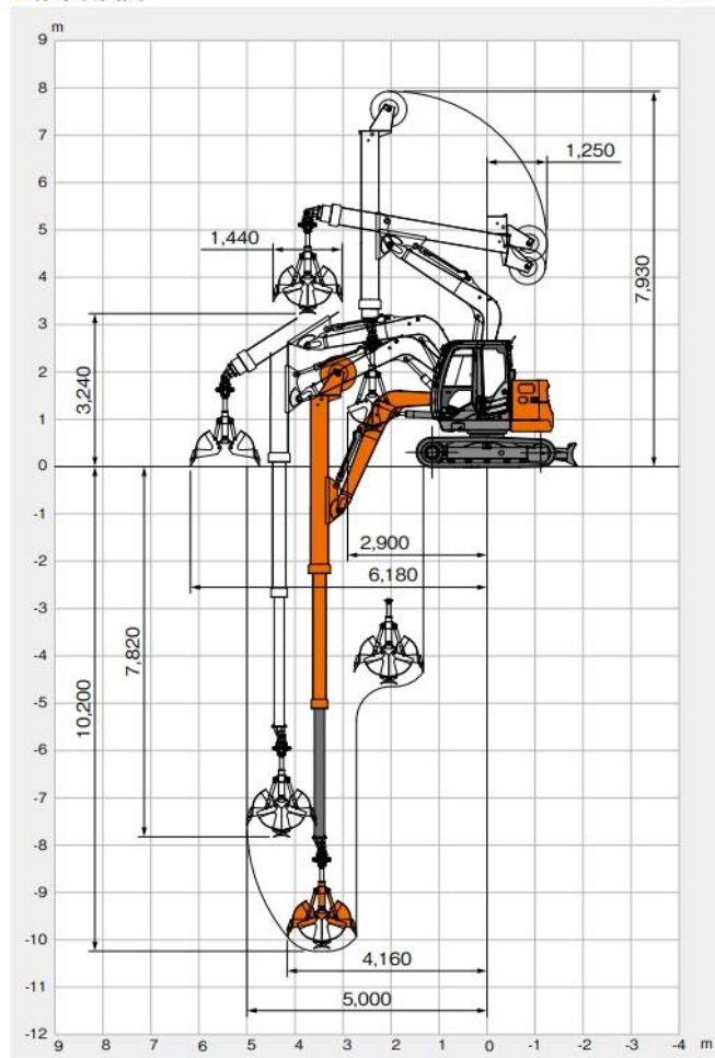
■作業範囲図
