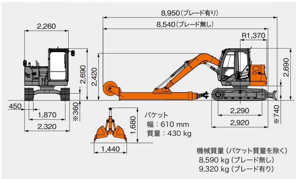
■寸法図および輸送範囲図
